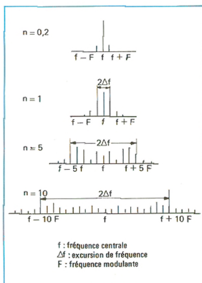
Figure 8 - Spectres d'une onde modulée en fréquence
