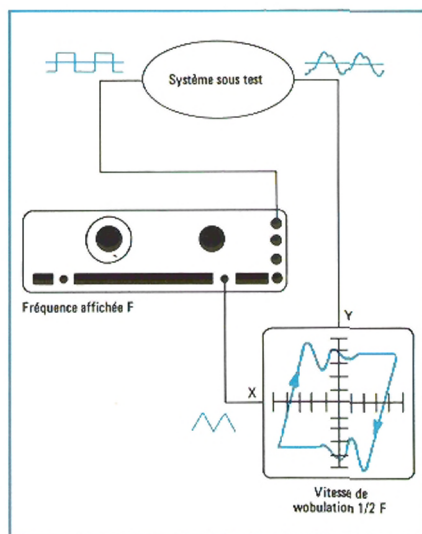
Fig. 2 Exemple d'application du FG 600 : Mesure de réponse transitoire
