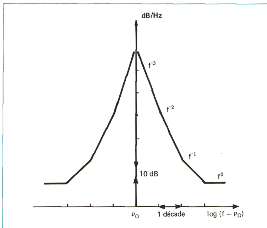
Fig. 1 - Pentes du spectre RF
