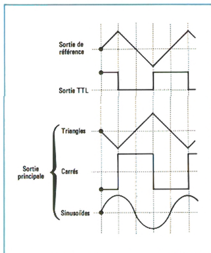
Fig. 1 Relation de phase entre les différentes sorties du FG 600.
