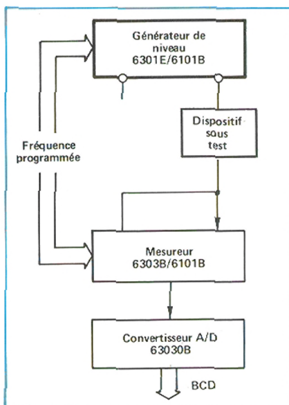
Figure 2 - Mesure directe de l'insertion d'un quadripôle actif ou passif.
