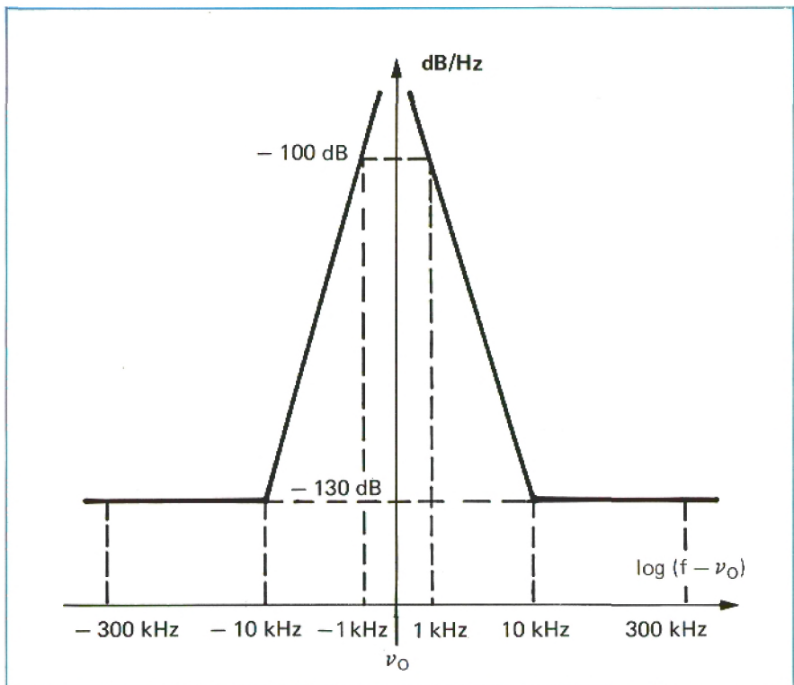
Fig. 3 - Exemple de spectre RF
