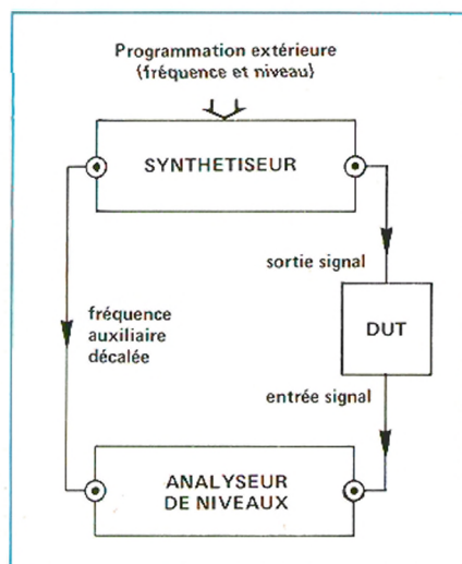
Fig. 2 - Mesures avec oscillateur suiveur
