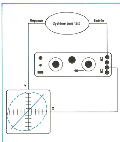
Exemple d'application du VPO 602 : Mesure de déphasage
