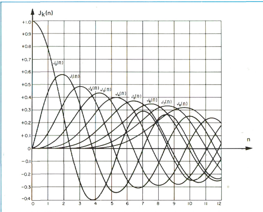
Figure 6 - Représentation graphique des fonctions de Bessel
