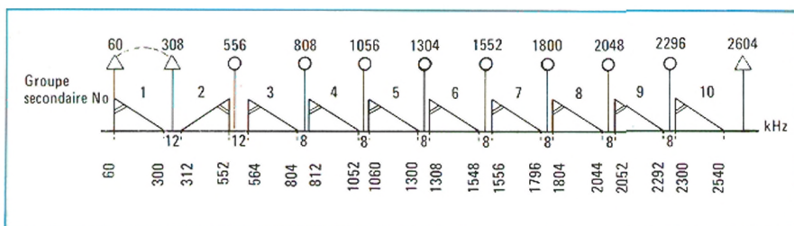
Fig. 5 - Plan de fréquence des groupes secondaires
