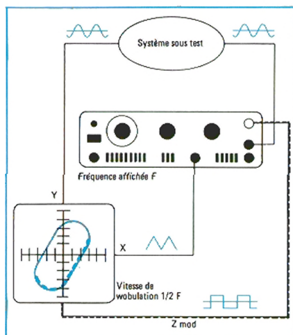
Fig. 2 - Exemple d'application de FG 601 : Mesure de réponse en fréquence
