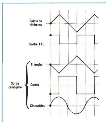
Fig. 1 - Relation de phase entre les différentes sorties du FG 601.
