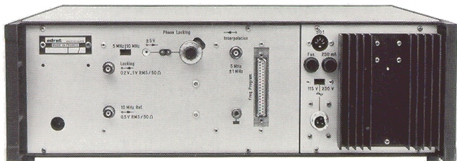
vue arrière du 3300 A
