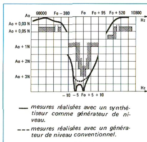
Fig. 4 - Réponse d'un filtre
