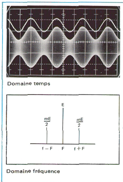
Fig. 2 - Modulation AM
