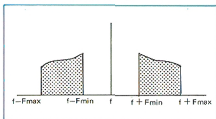
Figure 3 - Bandes latérales en modulation AM
