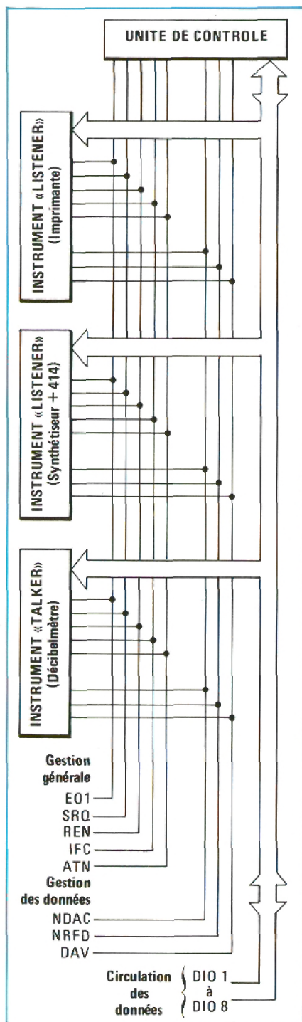
Fig. 3 - Principe de la voie omnibus bidirectionnelle IEC.
