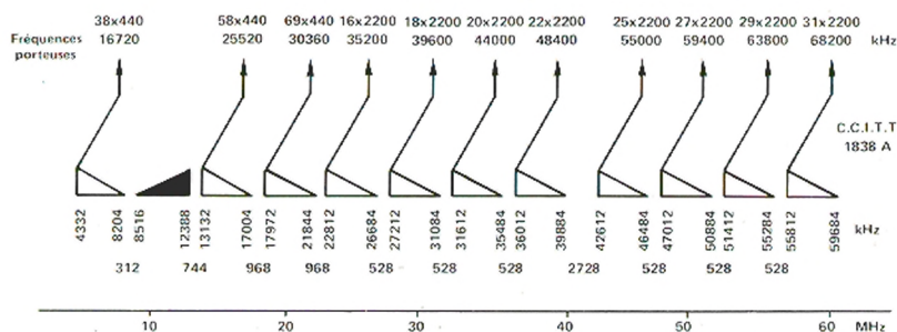
Figure 1 - Répartition des fréquences transmises pour des systèmes à 40 MHz et 60 MHz sur paires coaxiales 2,6/9,5 mm.
