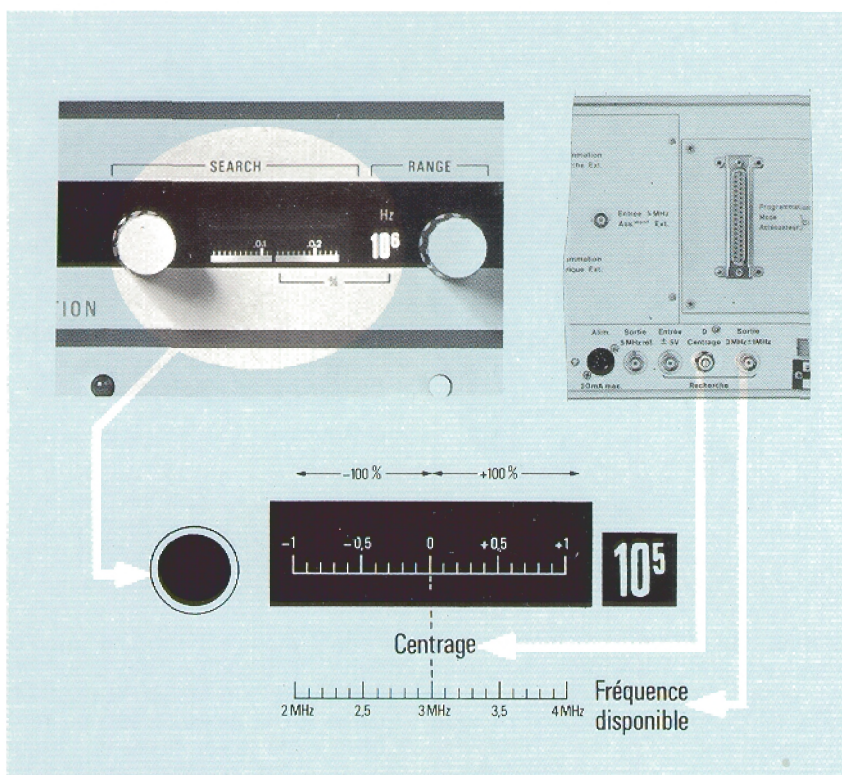
Figure 10 - Interpolation de fréquence
