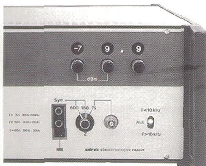
Détail du choix des impédances de sortie.
